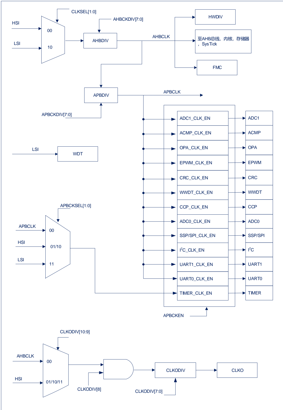
图 3-2: 时钟控制框图
