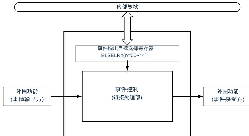
图19-1 EVENTC的框图
