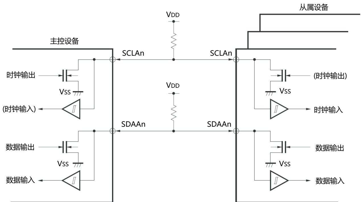
图16-12 引脚结构图
