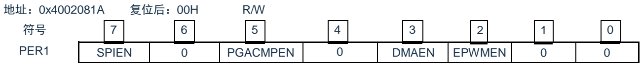
图12-3 外围允许寄存器1 (PER1) 的格式
