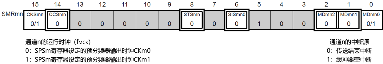
图14-313线串行I/O (SSPI00、SSPI01、SSPI10、SSPI11、SSPI20、SSPI21) 主控接收时的寄存器设定内容例子
