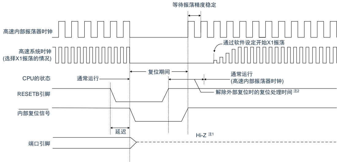
图23-2 RESETB输入的复位时序
