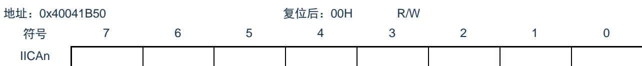
图16-3 IICAn移位寄存器n (IICAn) 的格式
