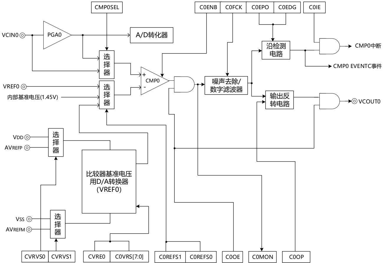
图12-1 比较器0的框图
