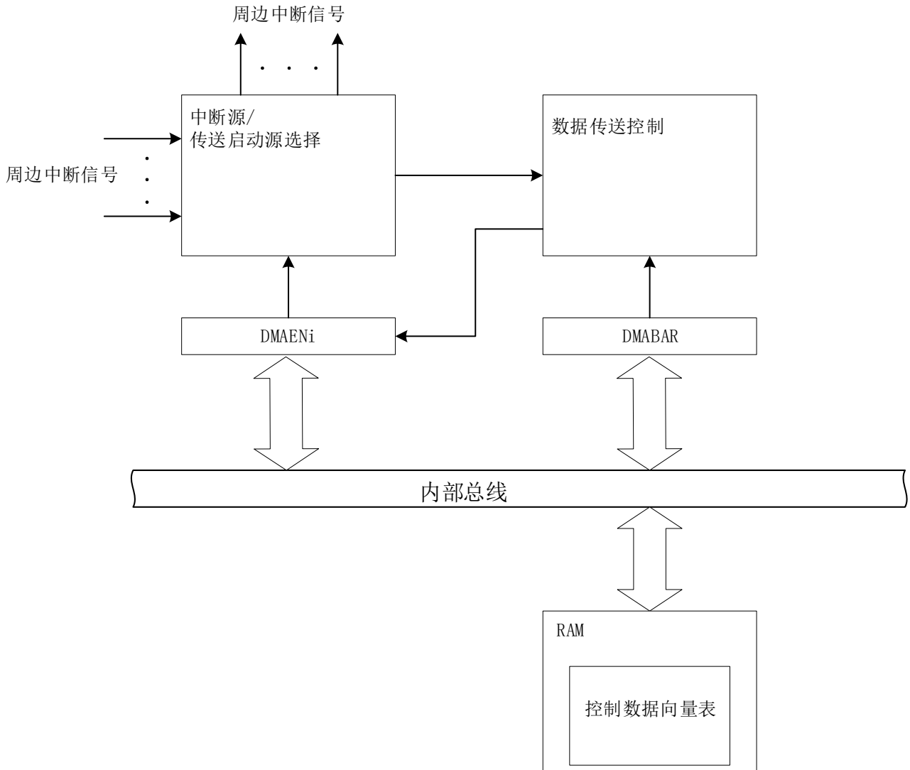
图18-1 DMA的框图
