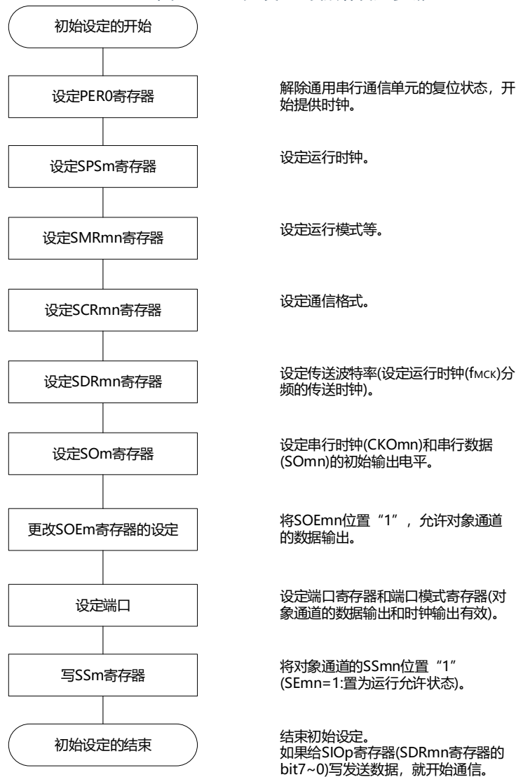
图14-24主控发送的初始设定步骤
