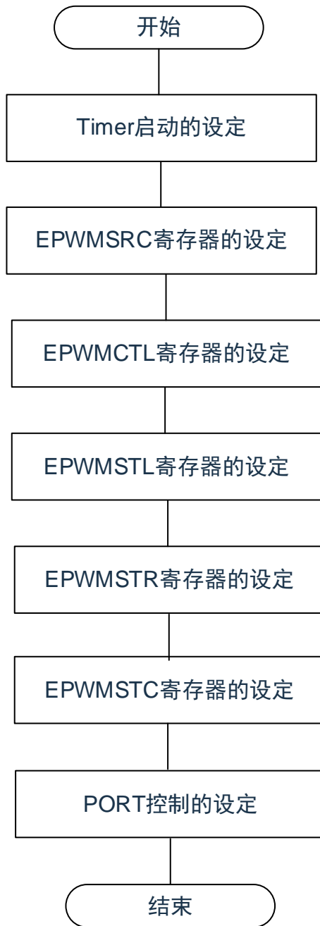
图6-7 寄存器的初始设定流程
