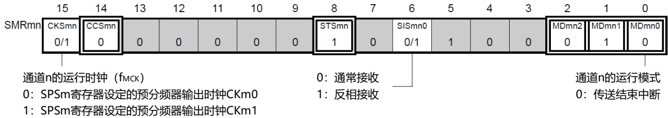
图14-104 UART (UART0~UART2) 的UART接收时的寄存器设定内容例子(1/2)
